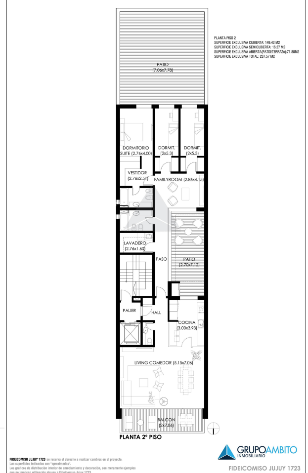
PLANTA 2º PISO - PLANTA TIPO DEL 3 - 9 PISO. DEPARTAMENTO DE 3 DORMITORIOS + FAMILYROOM
